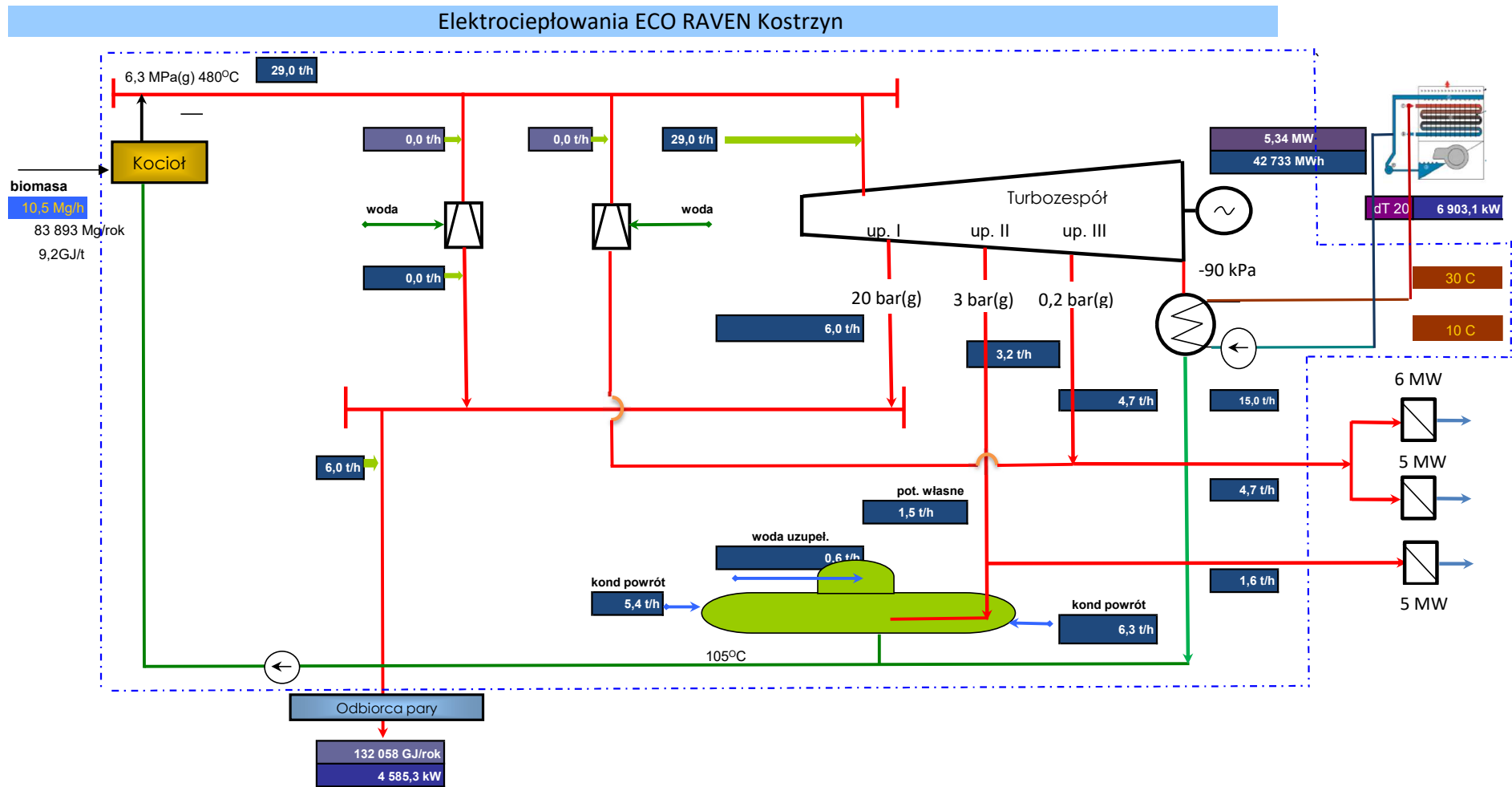
Załącznik 3. Schemat technologiczny - wartości średnioroczne
